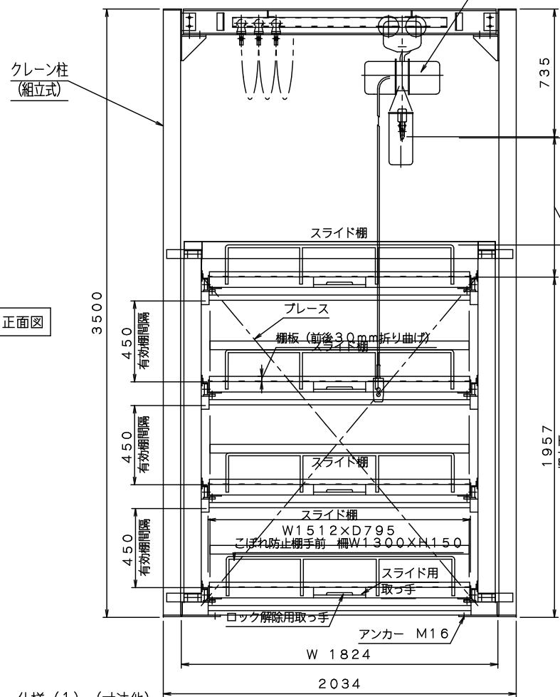
仕様 (1) (寸法他)
