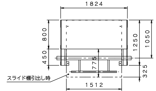
上面図
