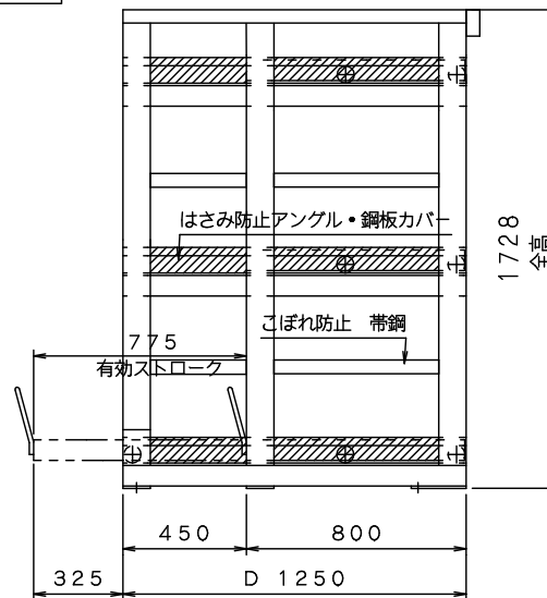
側面図
