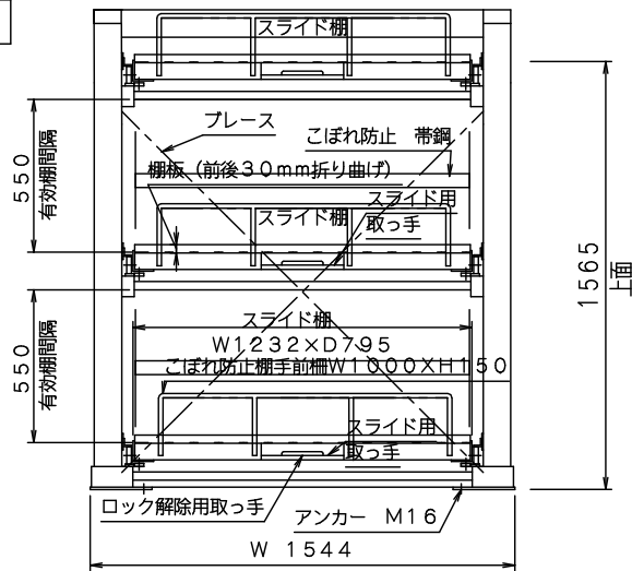
正面図
