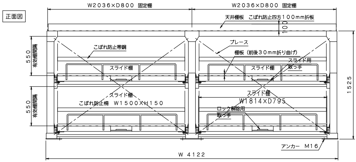
仕様(1) (寸法他)
