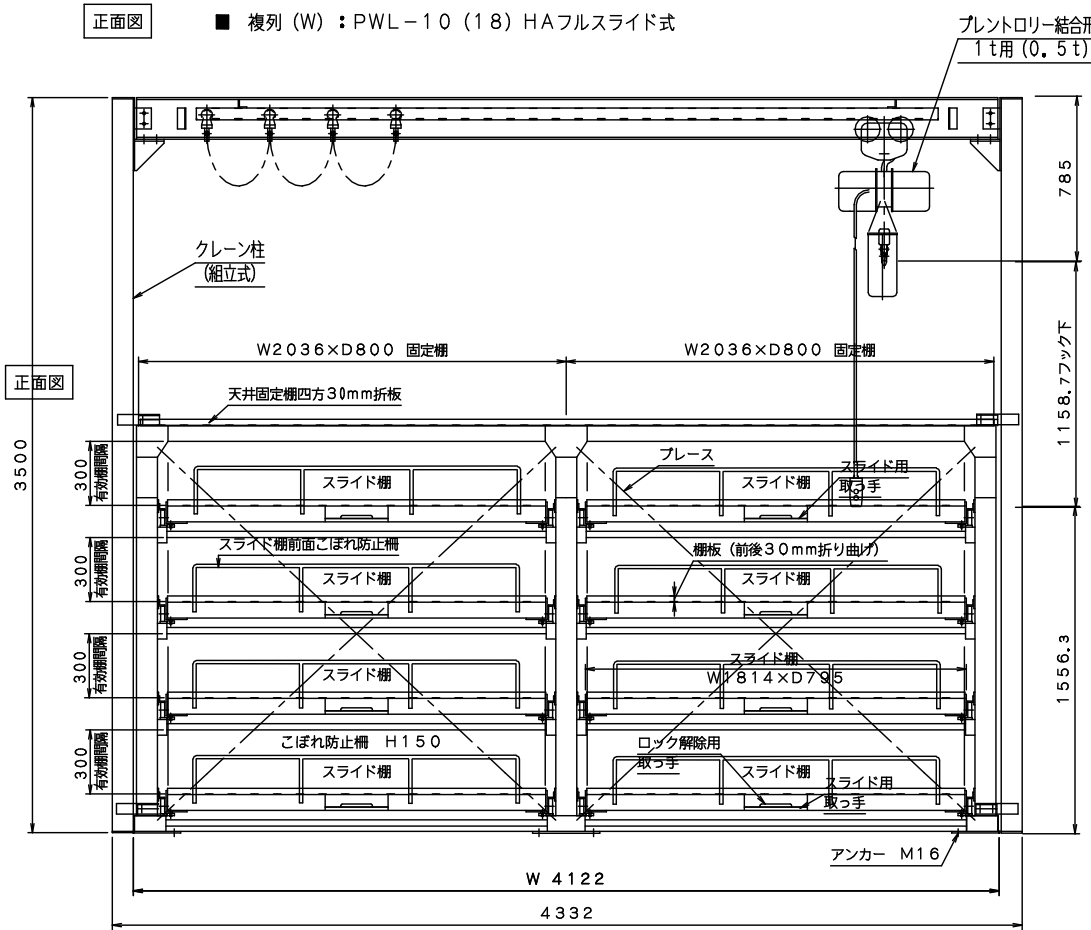
仕様 (2) (寸法他)
