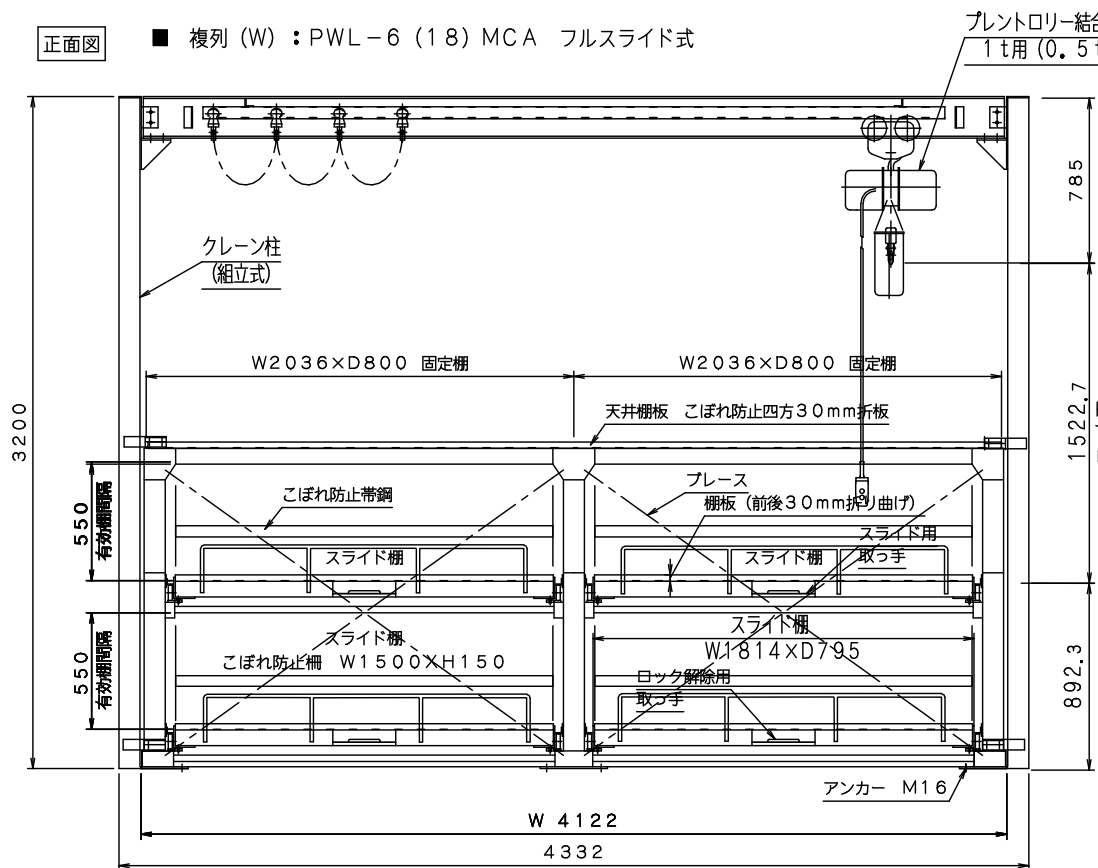
仕様 (2) (寸法他)
