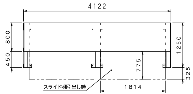
上面図 1/2スケール
