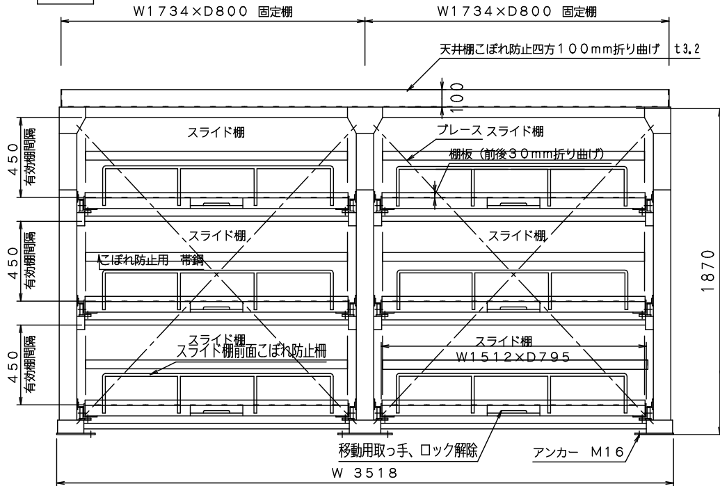
正面図
