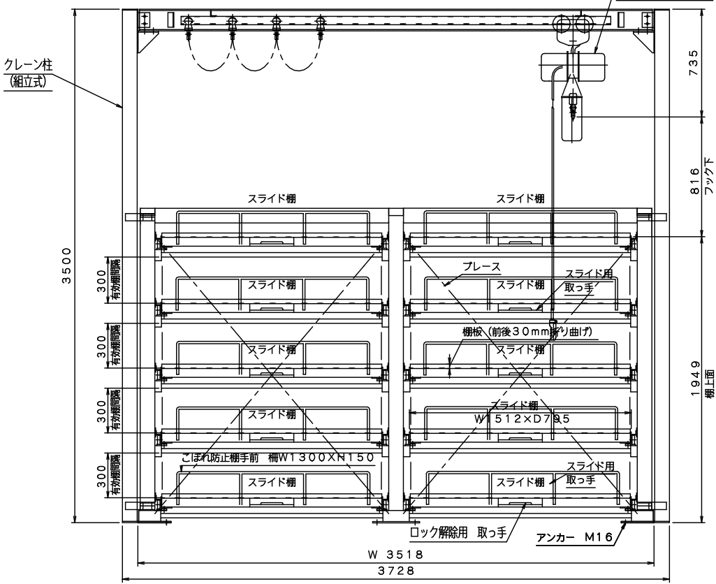
仕様 (2) (寸法他)
