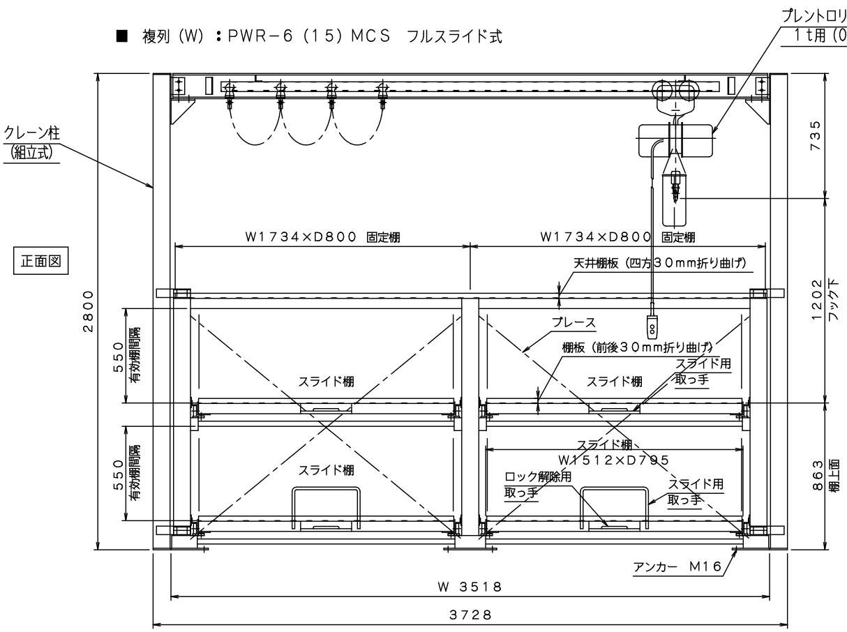
仕様 (1) (寸法他)
