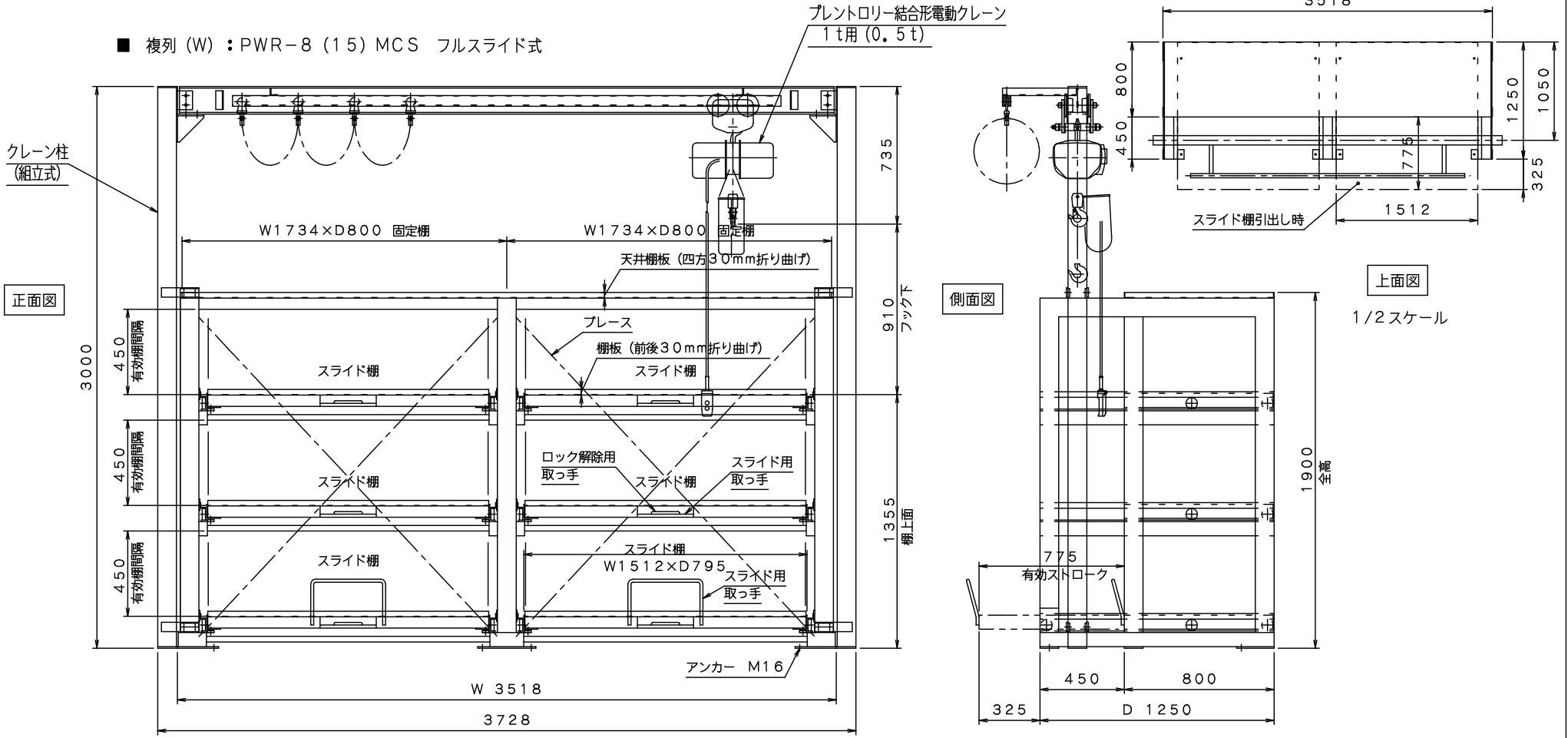
仕様 (1) (寸法他)
