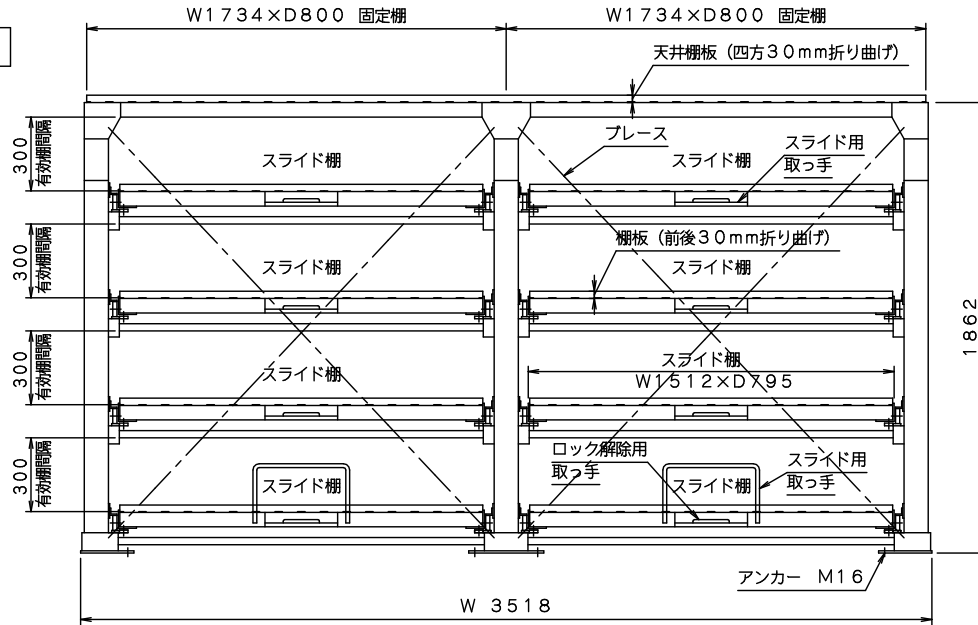
正面図
