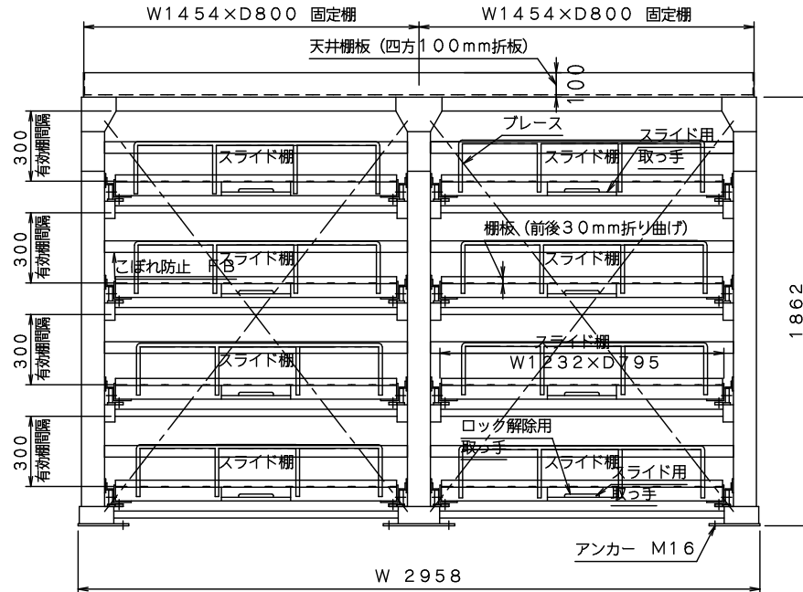
正面図
