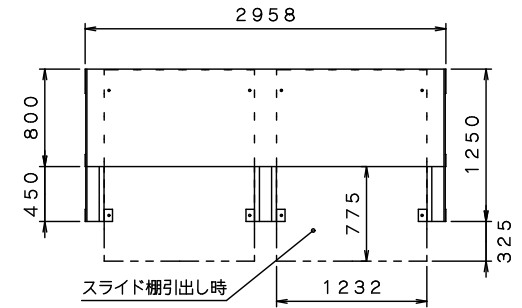
上面図 1/2スケール
