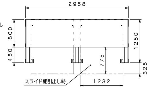
上面図
