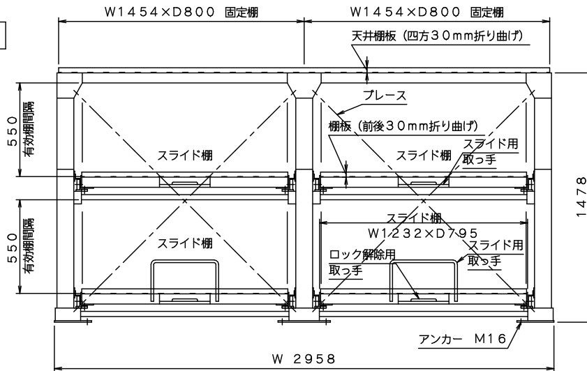
正面図
