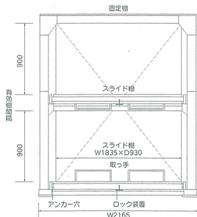
■単列 (S) : KS-3(5001) フルスライド式 [正面図]
