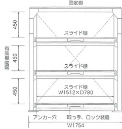
■単列 (S) : ESR-4(1102) フルスライド式 [正面図]
