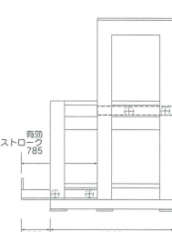
■単列・複列 [側面図]
