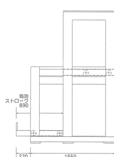
■単列・複列 [側面図]
