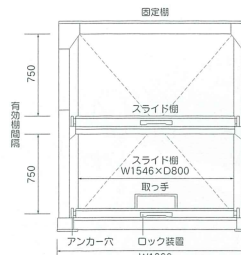
■単列 (S) : GS-3(3501) フルスライド式 [正面図]
